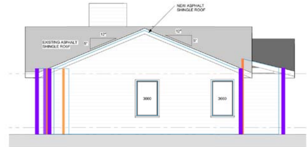
Right Elevation
